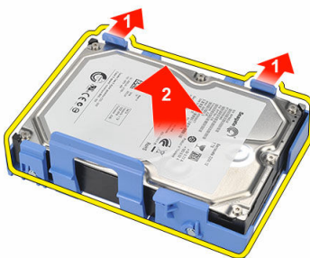
6. דחף את שתי הלשוניות מחוץ לכונן הקשיח והרם את הכונן הקשיח מתושבת הכונן הקשיח.
