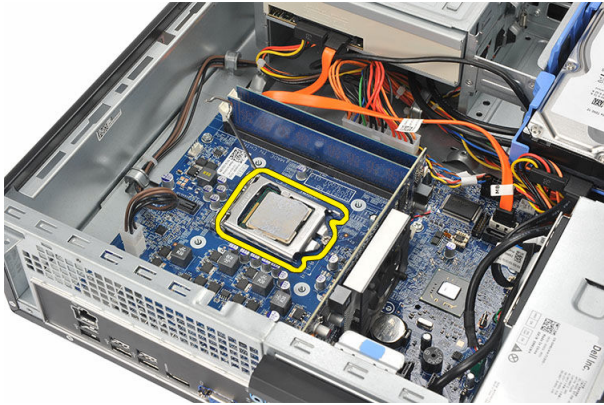
8. הרם את המעבד כדי להסירו מהשקע ולאחר מכן הנח אותו באריות הגנה מפני חשמל סטטי.
